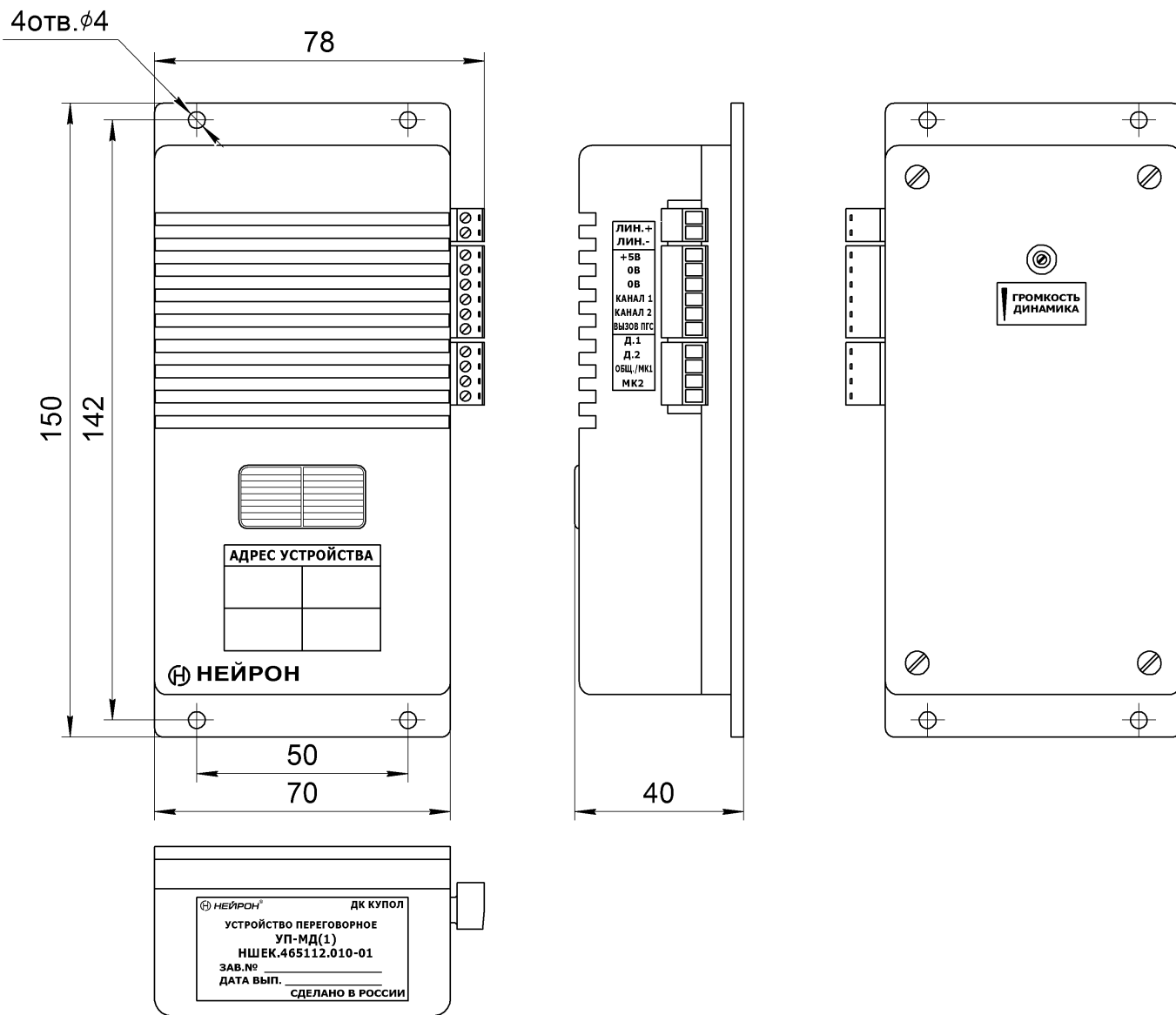
Рис.1 Внешний вид Устройства переговорного УП-МД(1) НШЕК.465112.010-01
